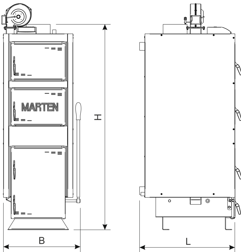
Малюнок 1 – Габаритне креслення котла типу Marten Comfort
